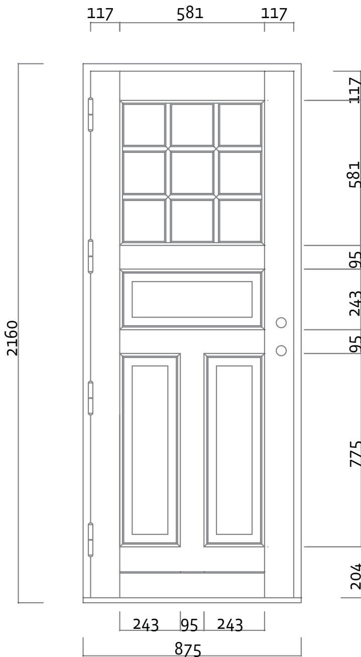
BD30 Fyldningsdør
