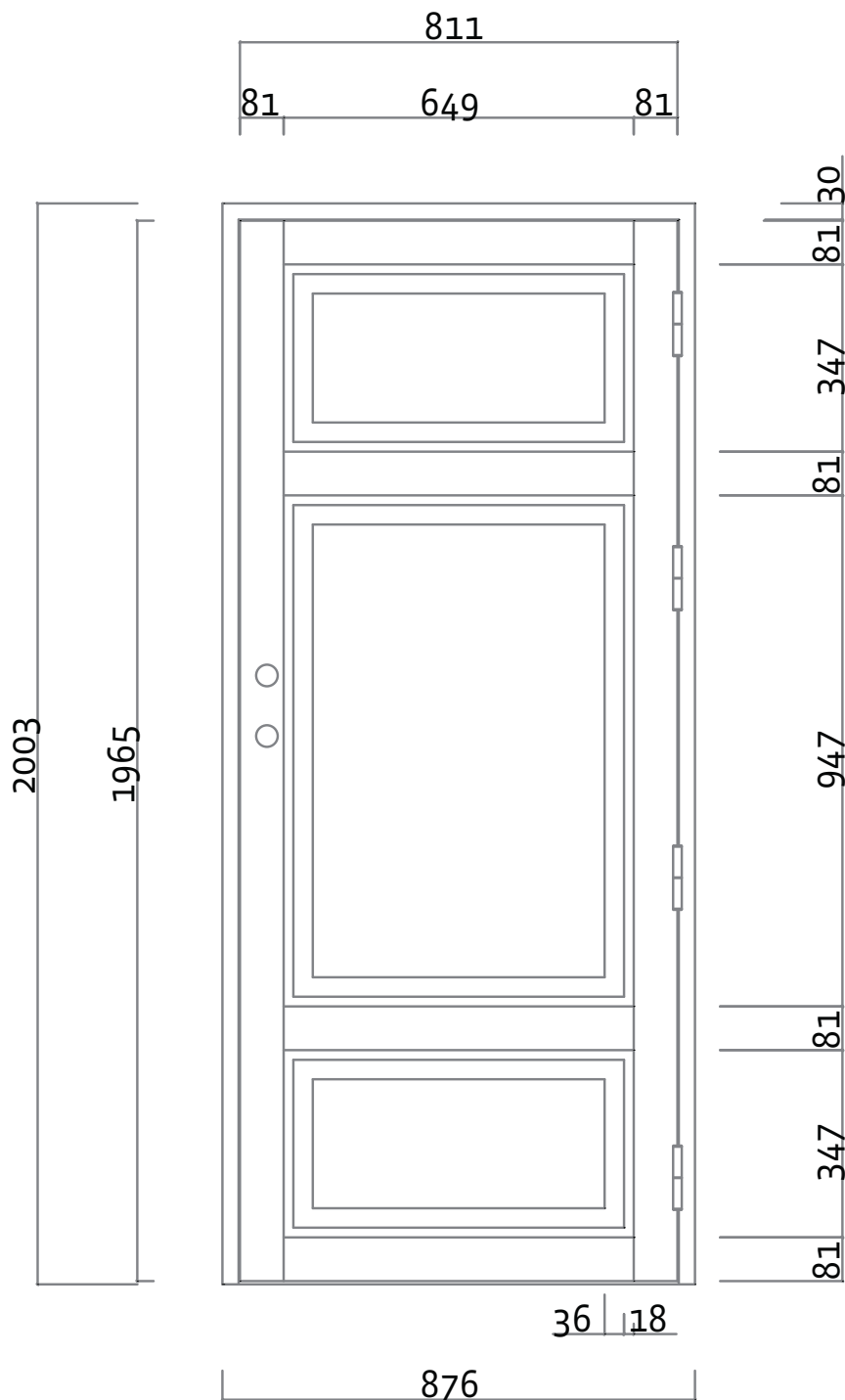
BD30 Fyldningsdør type D 012
