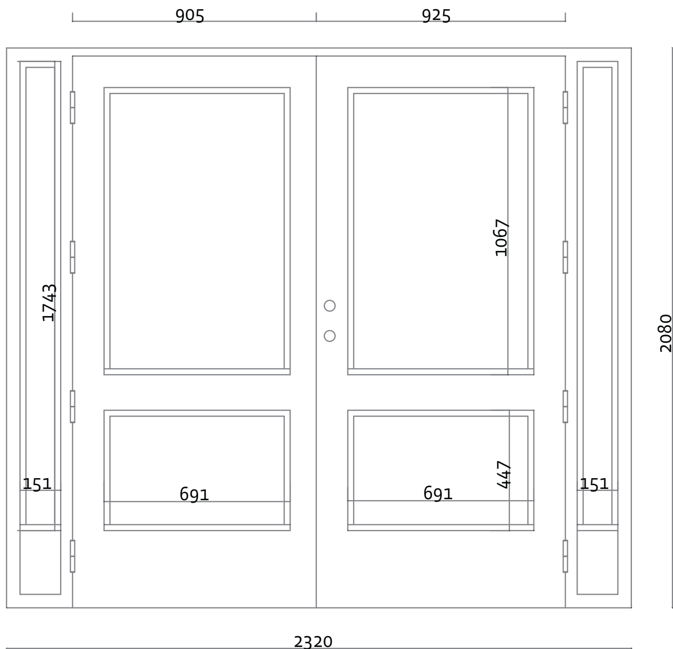
BD 60 Højregående Dobbeltdør m. sidepartier
