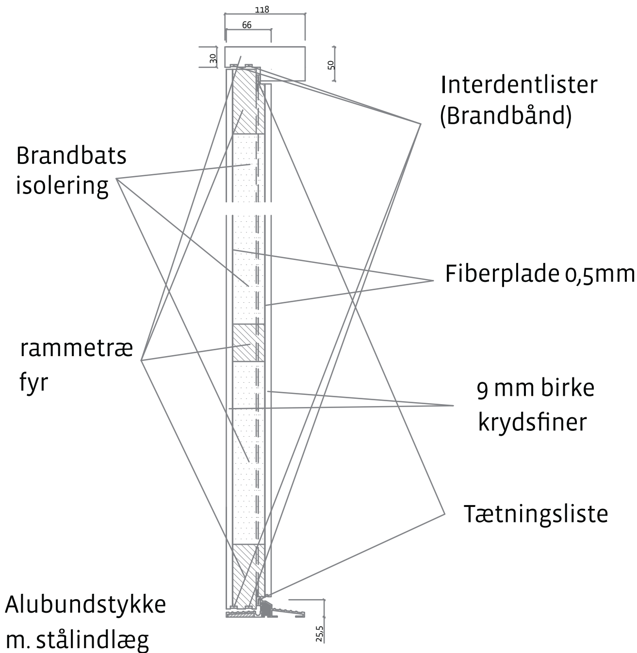
BD 60 snit massiv dør
