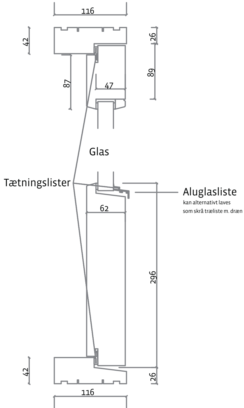
Snedkerdør snit
